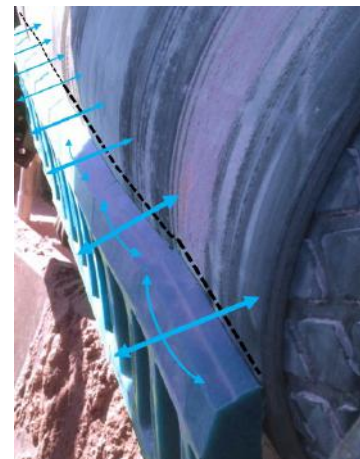
Die Multi-Klingen des RacloFlex Z 2 folgen dem Profil des Bandes und passen sich perfekt an.
